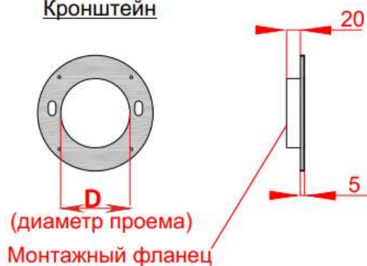
Кронштейн
